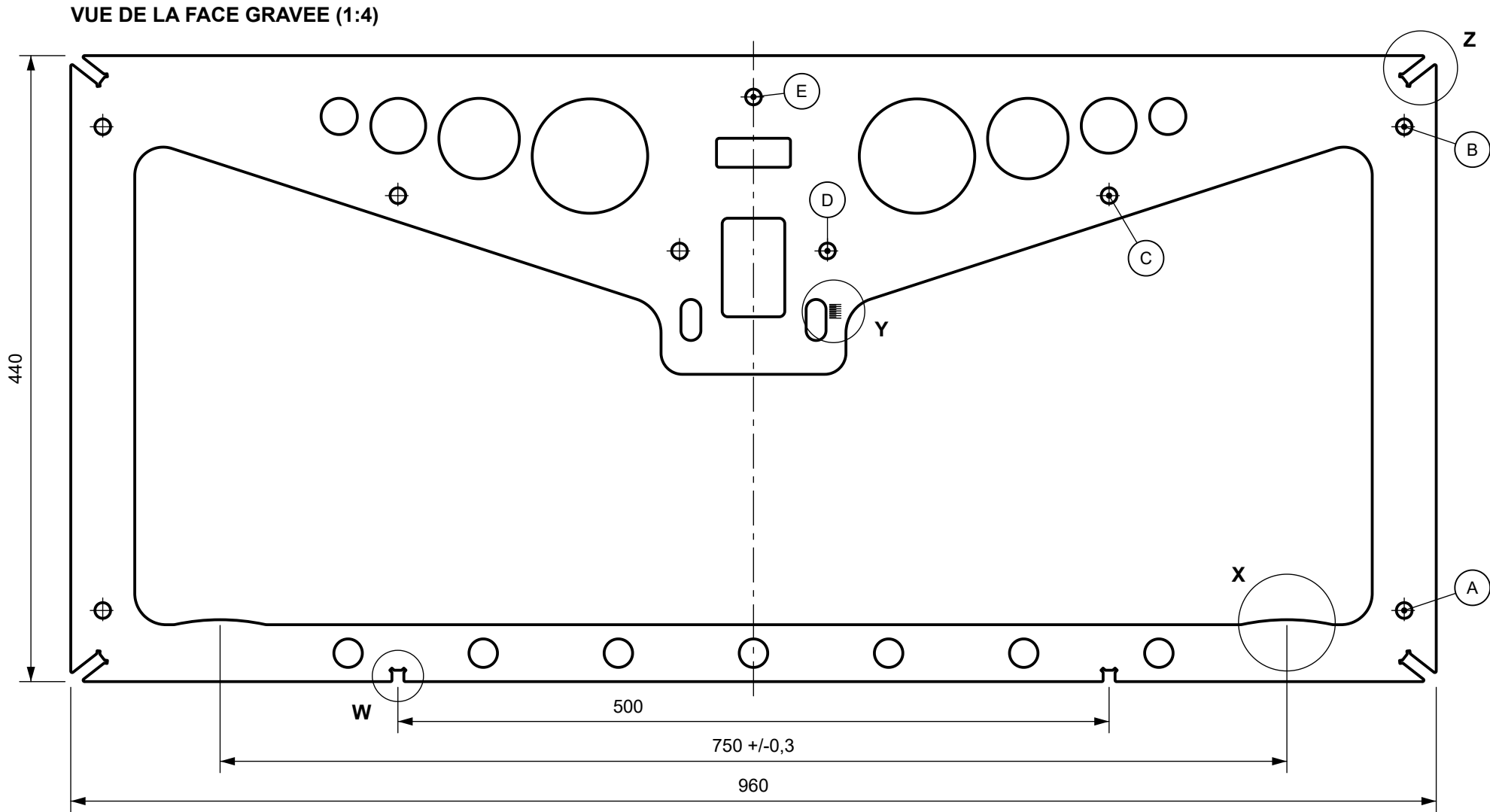
PERCAGES (X depuis l'axe, Z depuis le chant bas)
