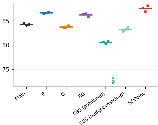
AdamW (lr 0.02)
