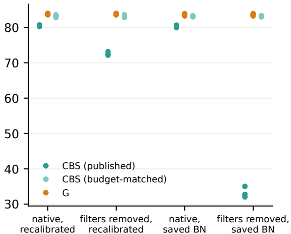
AdamW (lr 0.02)
