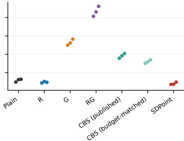
AdamW (lr 0.02)
