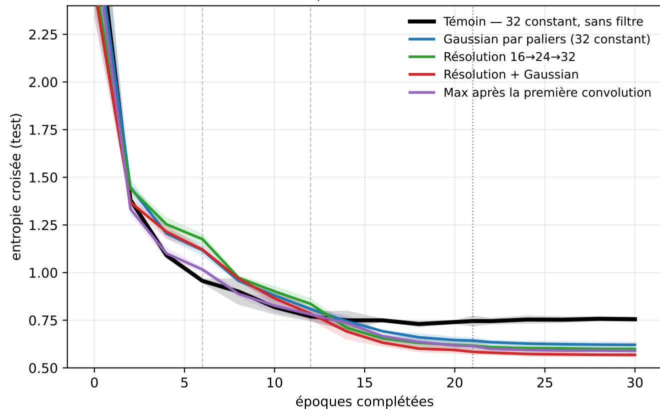
Entropie croisée de test
