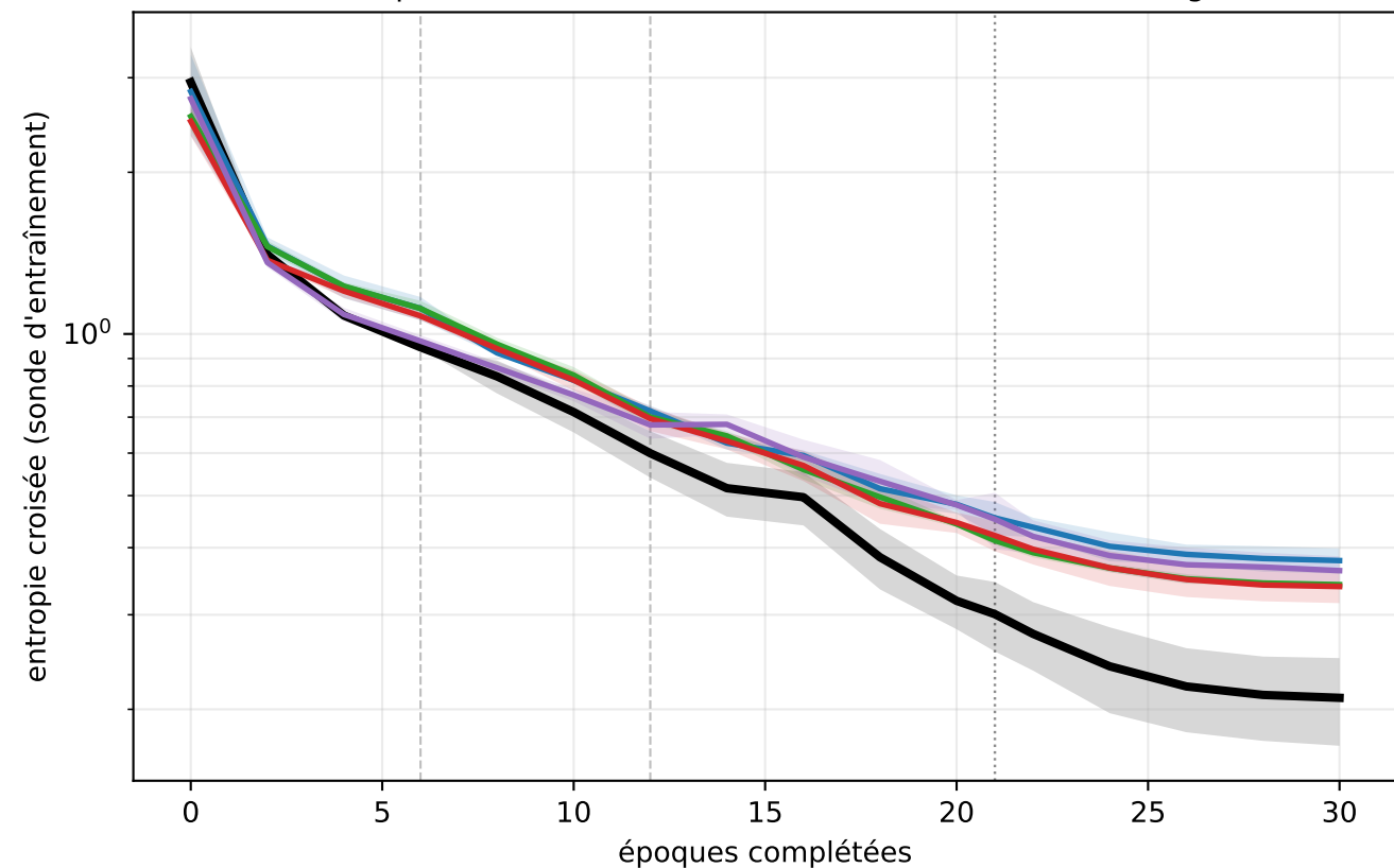
Entropie croisée sur la sonde d'entraînement (échelle log)
