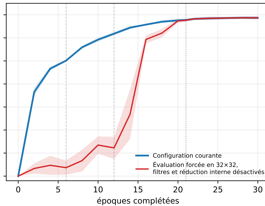
Résolution 16→24→32, sans filtre, Max après la première convolution
