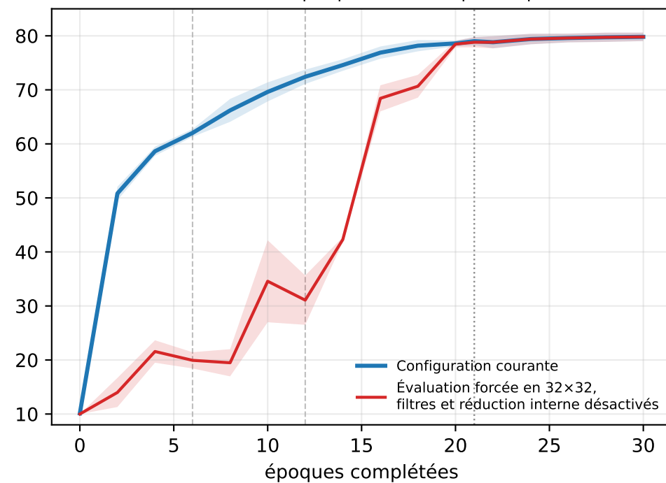
Résolution 16→24→32, Gaussian par paliers, Max après la première convolution
