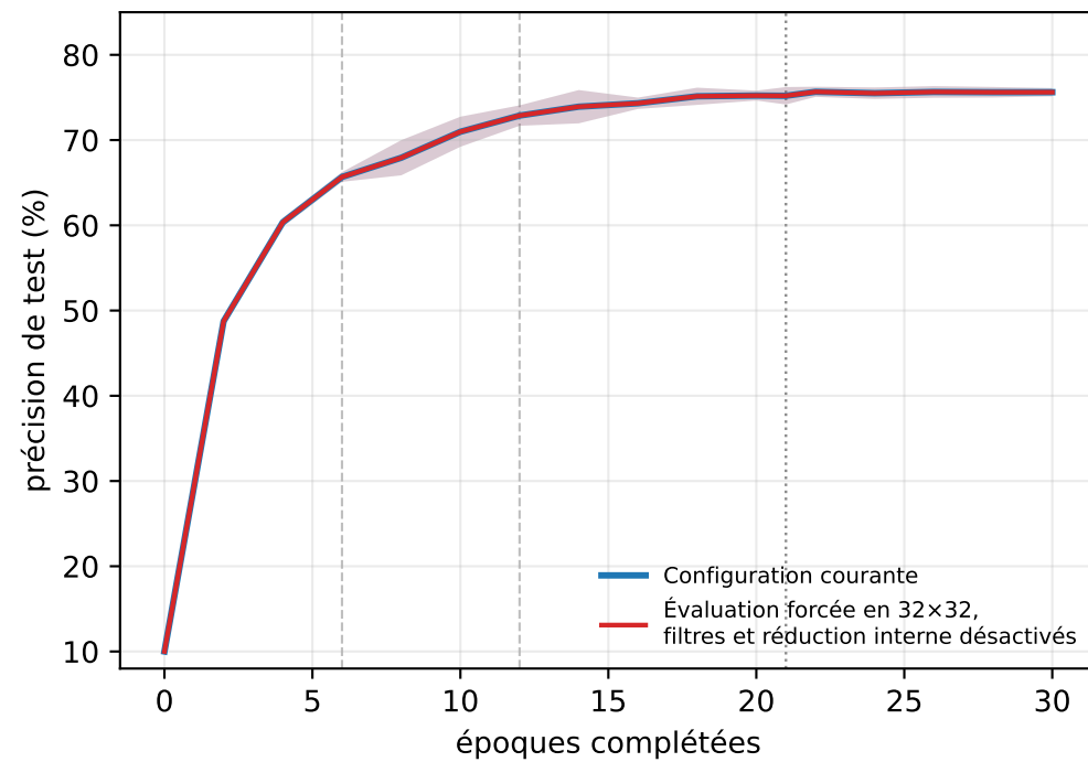
Résolution 16→24→32, Gaussian par paliers
