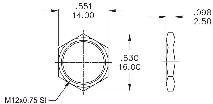
NUT
