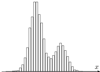
(d) Mixture
