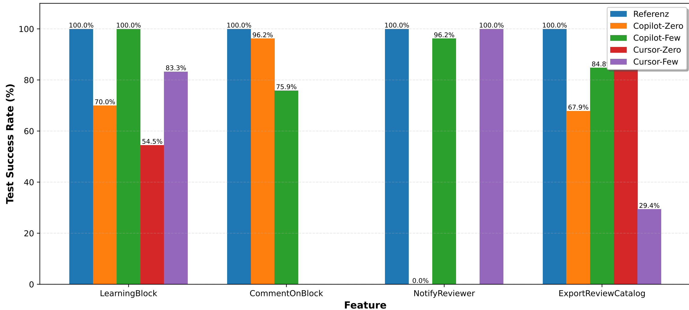
Test Success Rate nach Feature und Implementierungsvariante
