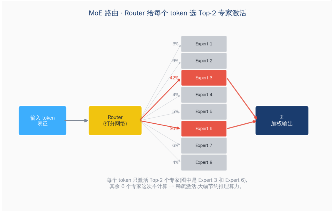
图 M7.1 · MoE 路由 · Router 给每个 token 选 Top-2 专家激活 (稀疏计算节省推理算力)
