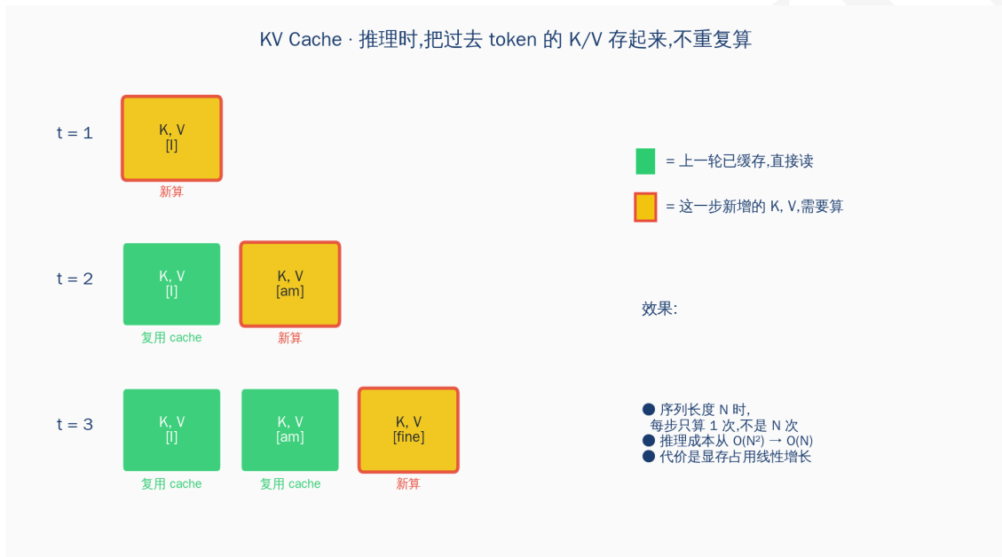
图 M3.5 · KV Cache 推理时复用过去 token 的 K/V \rightarrow O(N^2) \rightarrow O(N)
