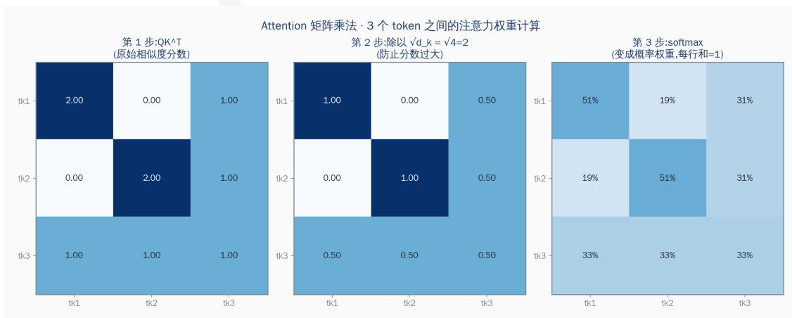
图 M3.3 · Attention 矩阵乘法三步 · QK \rightarrow 缩放 \rightarrow softmax 权重
