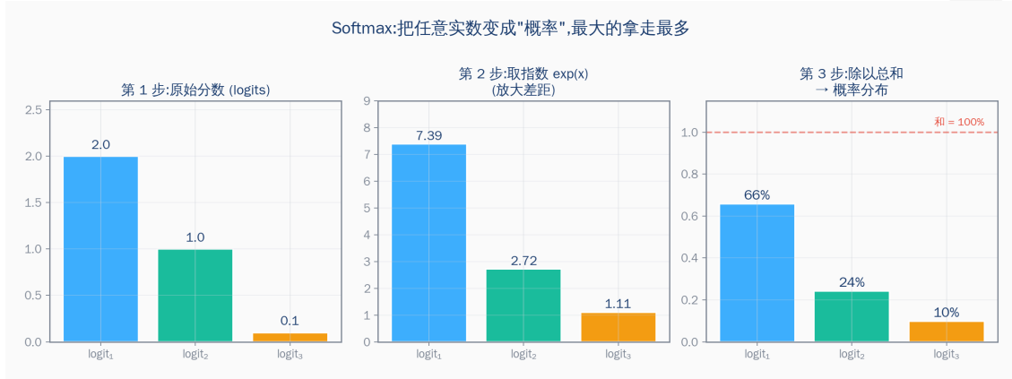
图 M3.2 · Softmax · 把任意实数变成概率 (放大差距 → 归一化)
