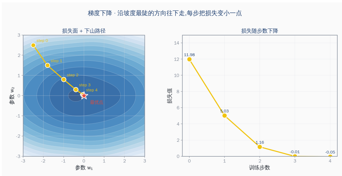
图 M4.1 · 梯度下降 · 沿坡度最陡的方向下山，每步把损失变小一点
