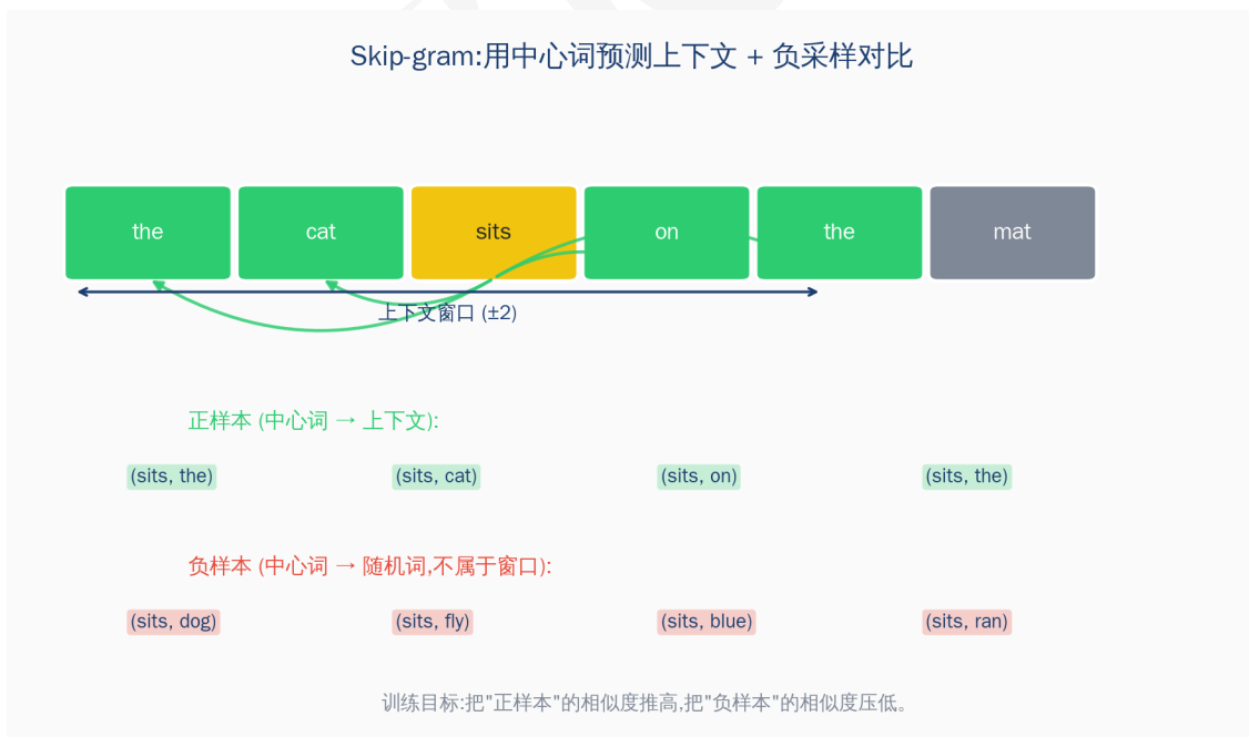
图 M2.1 · Skip-gram 训练范式 · 用中心词预测上下文 + 负采样对比
