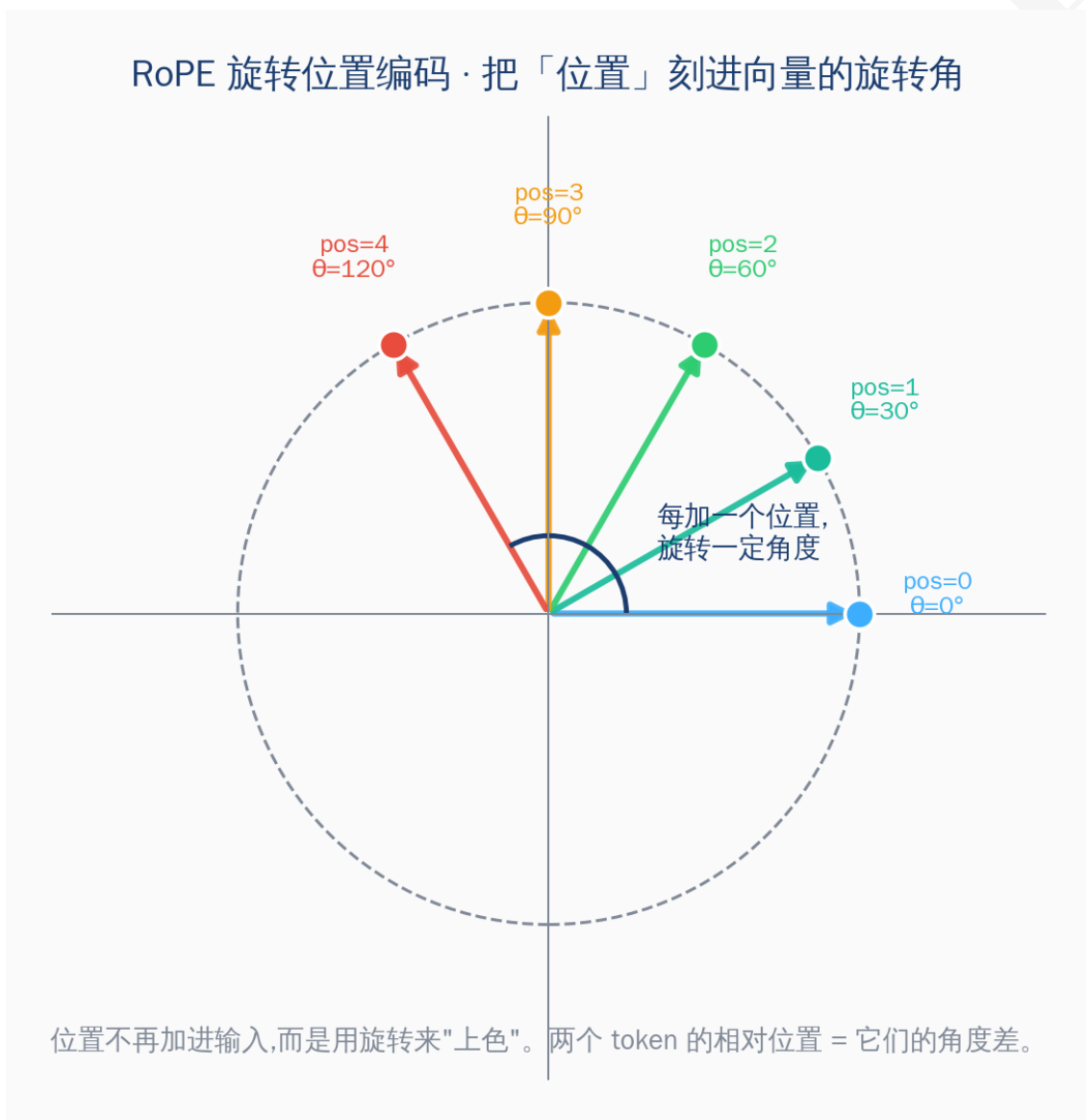
图 M3.4 · RoPE 旋转位置编码 · 把「位置」刻进向量的旋转角
