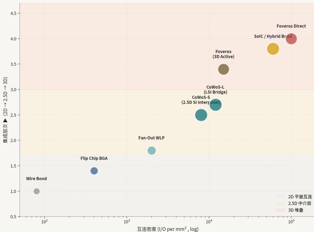
图 17.x 先进封装家族象限图: 互连密度 vs 集成层次
