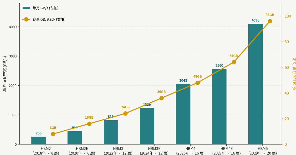
图 19.x HBM 高带宽内存代际演进 (容量 / 带宽 / 堆叠层数)
