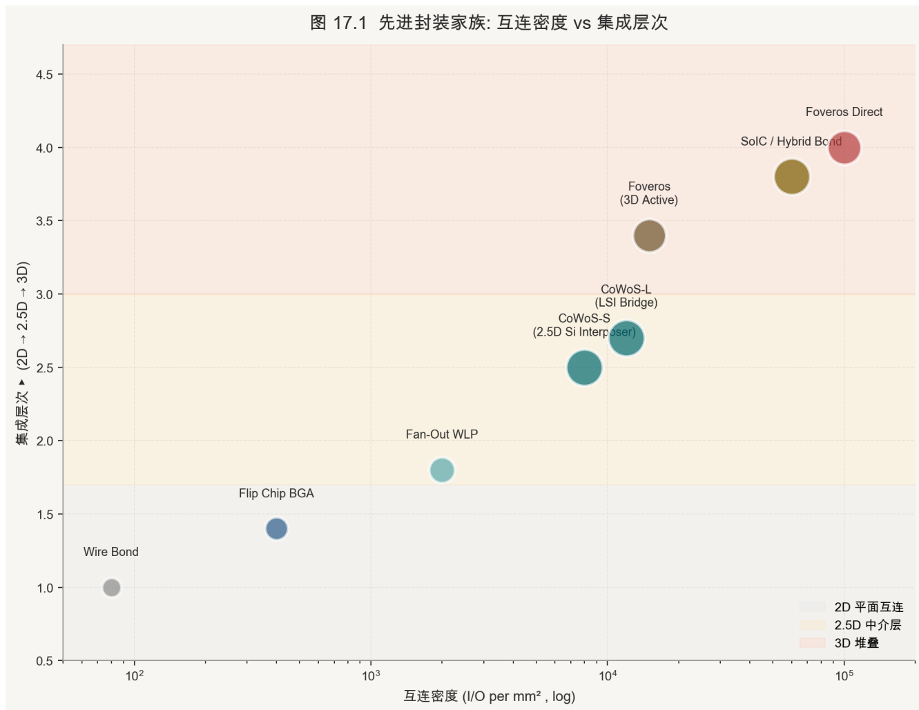
图 17.1 先进封装家族象限图: 互连密度与集成层次
