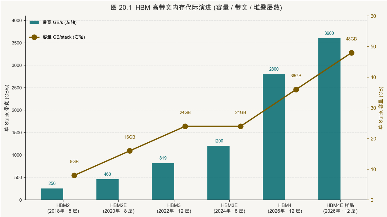
图 20.1 HBM 高带宽内存代际演进 (容量、带宽与堆叠层数)
