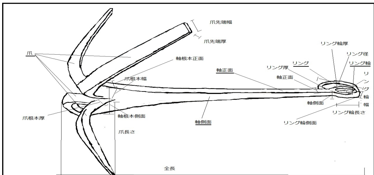
図1 四爪錨各部呼称 (銚子市青少年文化会館所蔵錨を元に自作)
