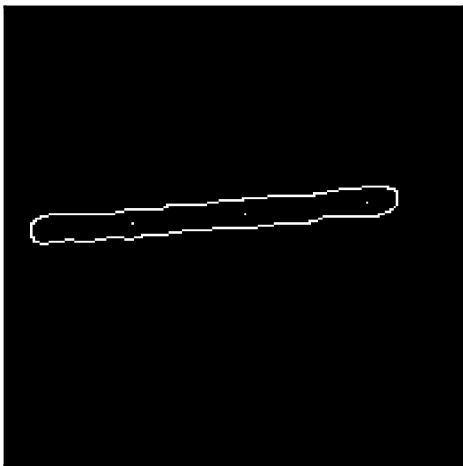
d. \sigma = 3
