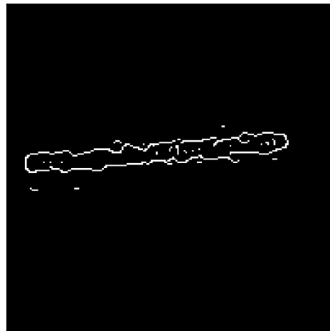
f. \sigma = 10
