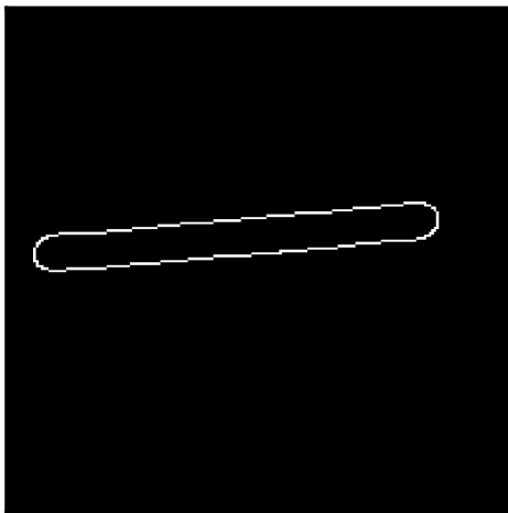
e. \sigma = 5
