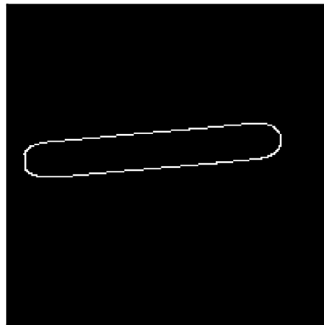
f. \sigma = 10
