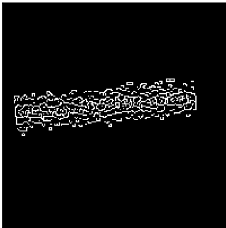
e. \sigma = 5
