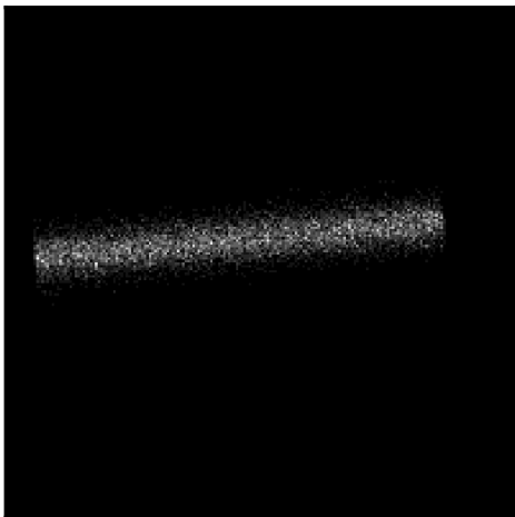
d. \sigma = 3
