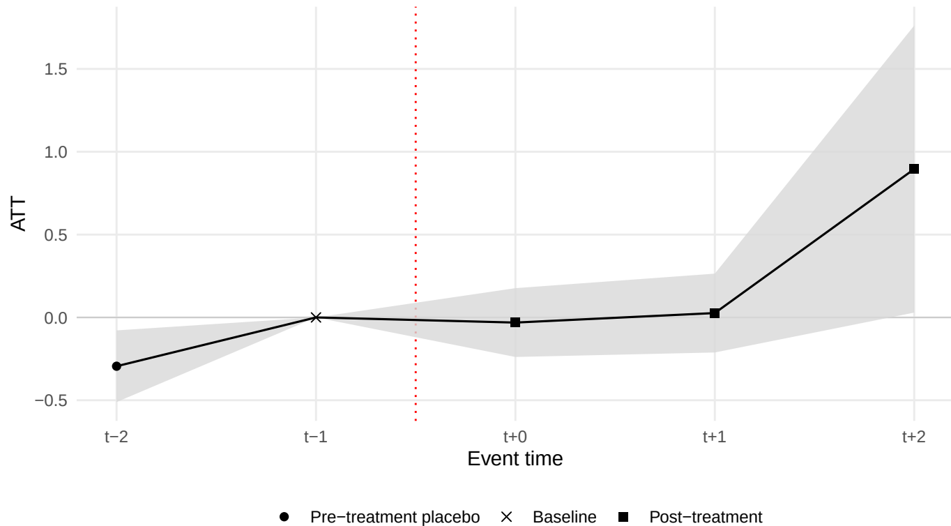
PanelMatch dynamic estimates – asinh_valore_aggiunto_w
