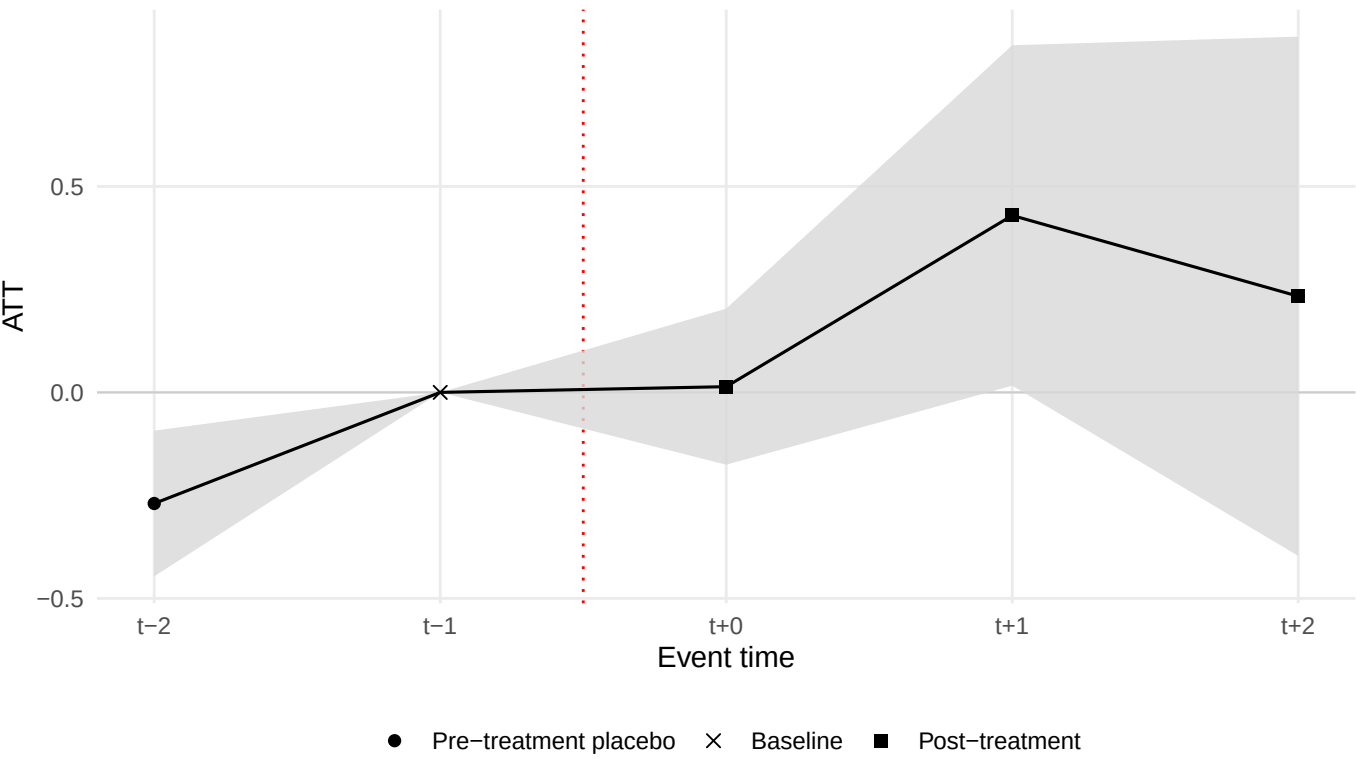
PanelMatch dynamic estimates – asinh_valore_aggiunto_w (Mahalanobis – 3 neigh
