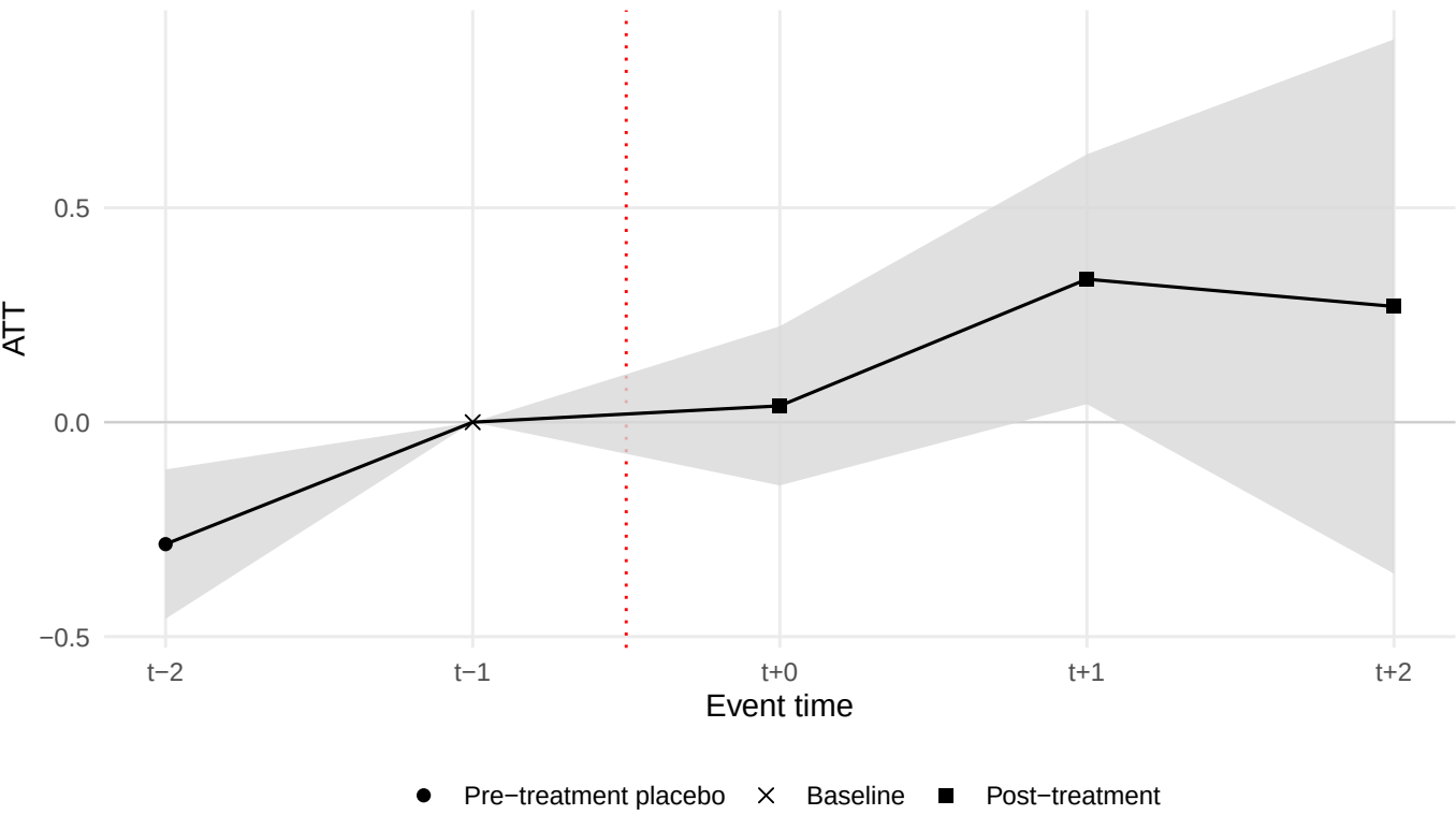
PanelMatch dynamic estimates – asinh_valore_aggiunto_w (Mahalanobis – 5 neigh
