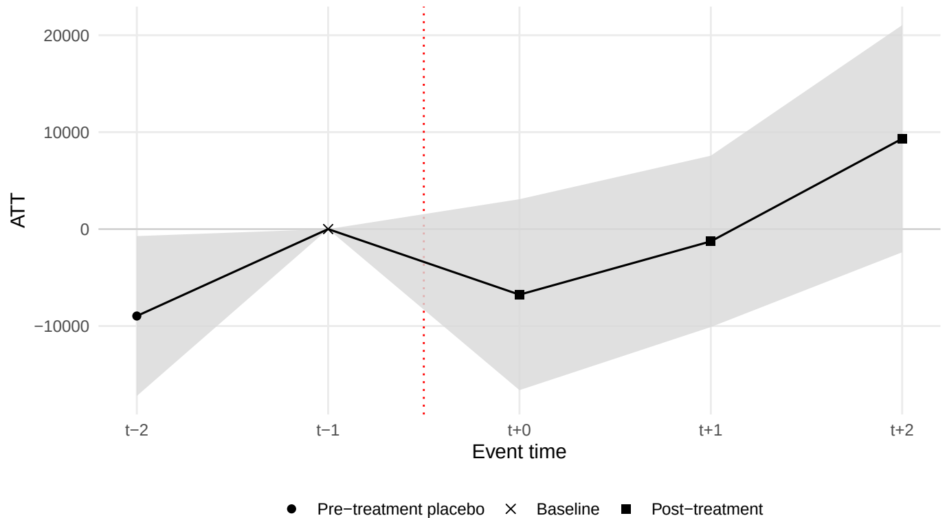
PanelMatch dynamic estimates – valore_aggiunto_w (Mahalanobis – 5 neighbo
