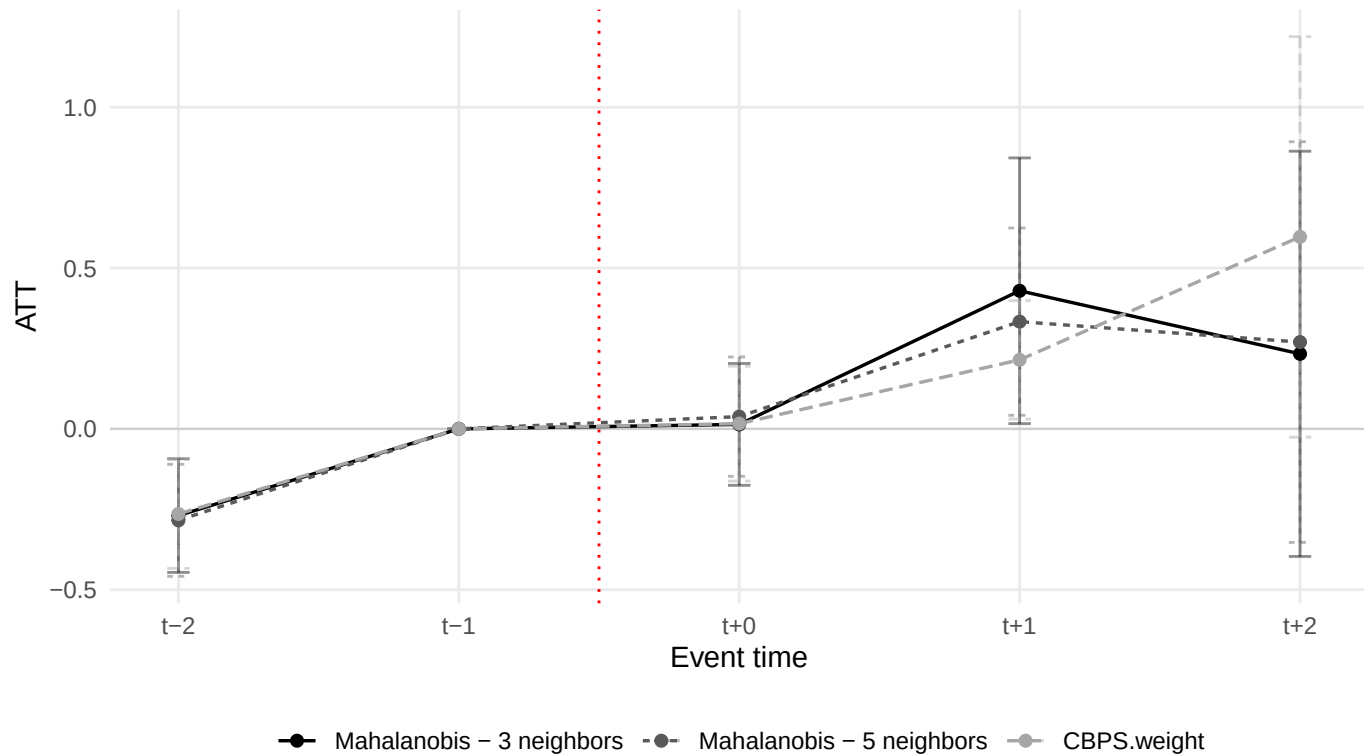
PanelMatch refinement comparison – asinh_valore_aggiunto_w
