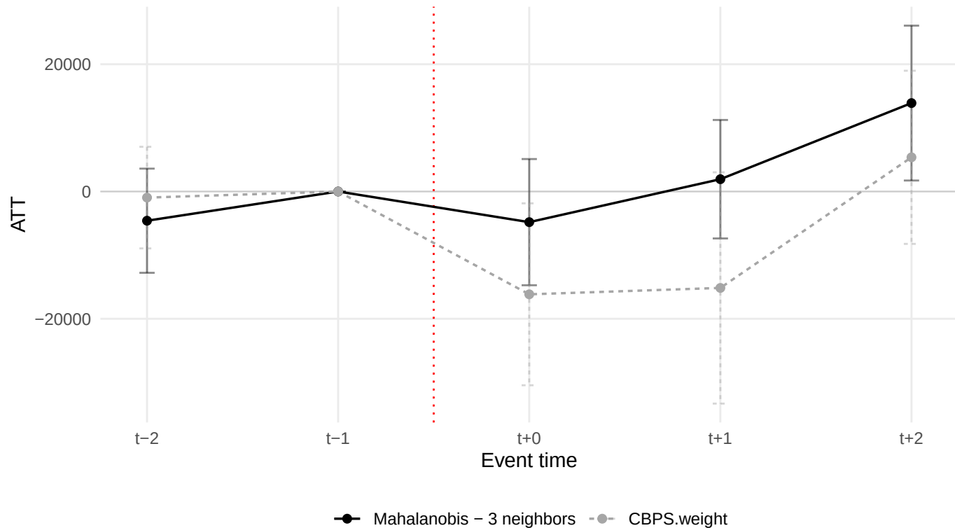
PanelMatch refinement comparison – valore_aggiunto_w
