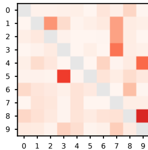
SVM
