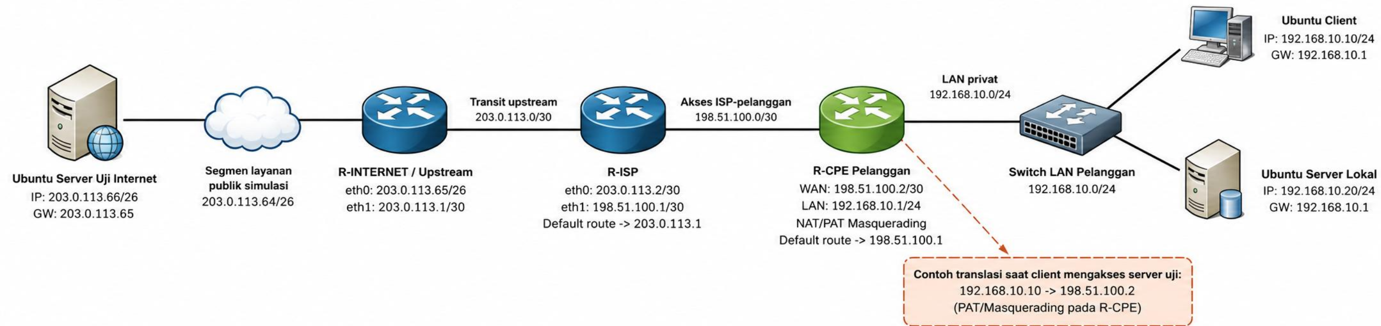
Gambar 3.1 Diagram Topologi Jaringan ISP dan Pelanggan
