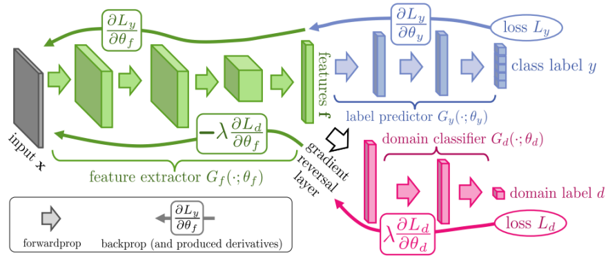
图 2 域对抗训练框架示意图。该框架包含三个主要组件：特征提取器（Feature Extractor）、标签预测器（Label Predictor）和域判别器（Domain Discriminator）。输入图像经过特征提取器得到特征表示，标签预测器基于特征进行类别预测（计算标签预测损失 L_y ），域判别器尝试区分特征来自源域还是目标域（计算域分类损失 L_d ）。通过梯度反转层（Gradient Reversal Layer），特征提取器学习到的特征既能够完成目标任务，又无法被域判别器区分来源，从而实现域不变特征学习。
