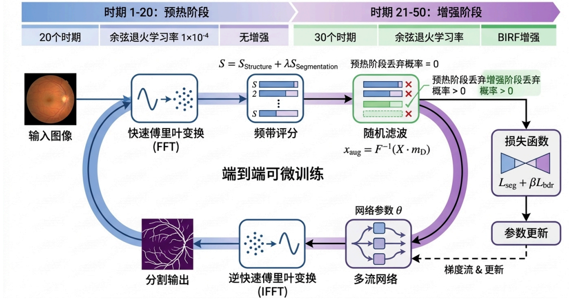
图 8 BIRF-SDG 训练流程示意图。训练过程分为预热阶段和增强阶段：前 20 个 epoch 仅使用原始图像训练，后 30 个 epoch 引入频带评分、随机滤波和多流网络联合优化。
