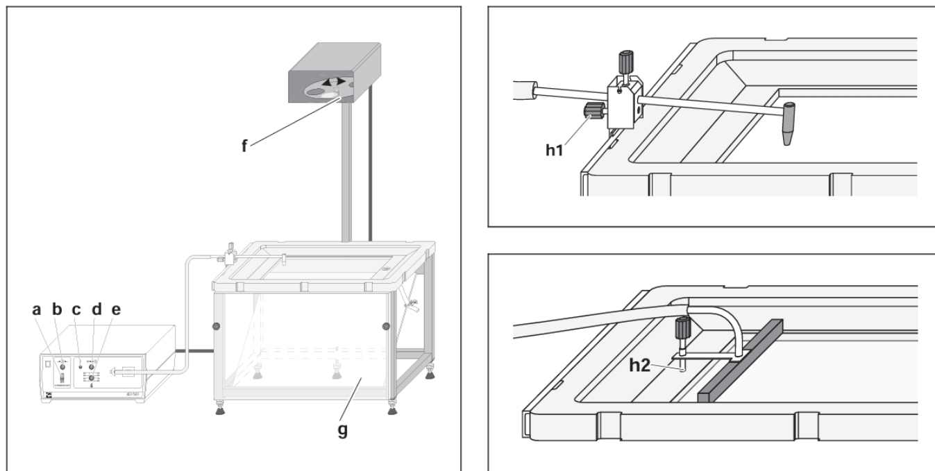
Figure 2: Cuve à ondes
