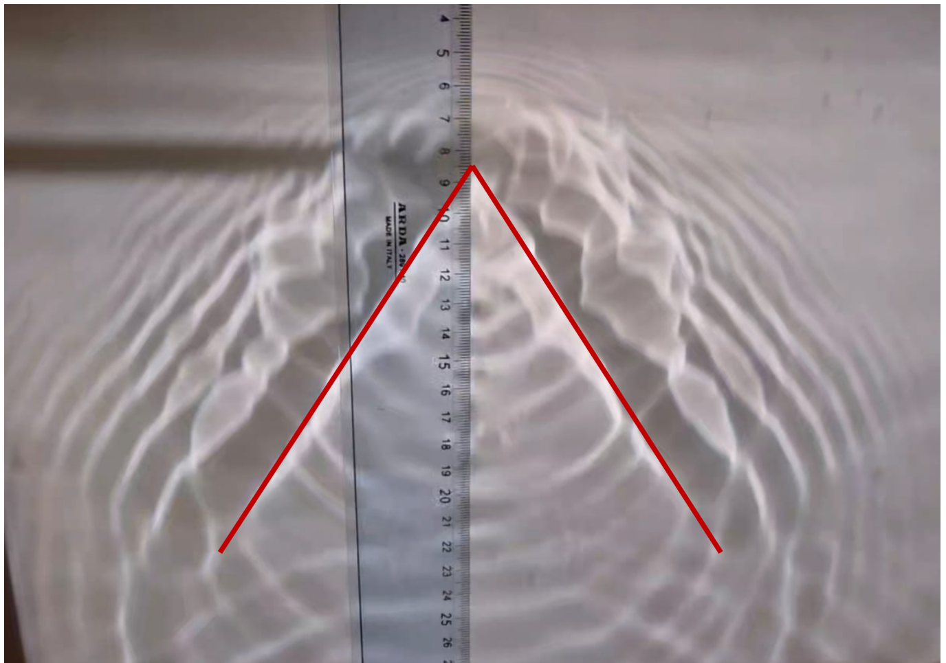
Figure 4: Cône de Mach
