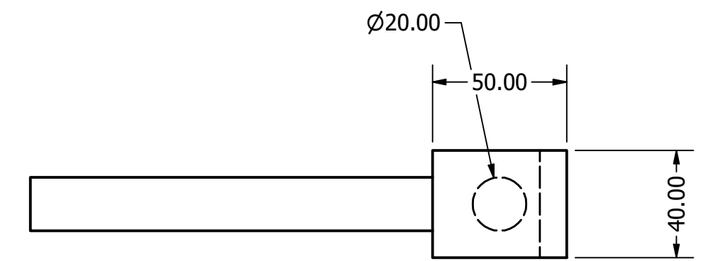
Clip SCALE 1 : 1
