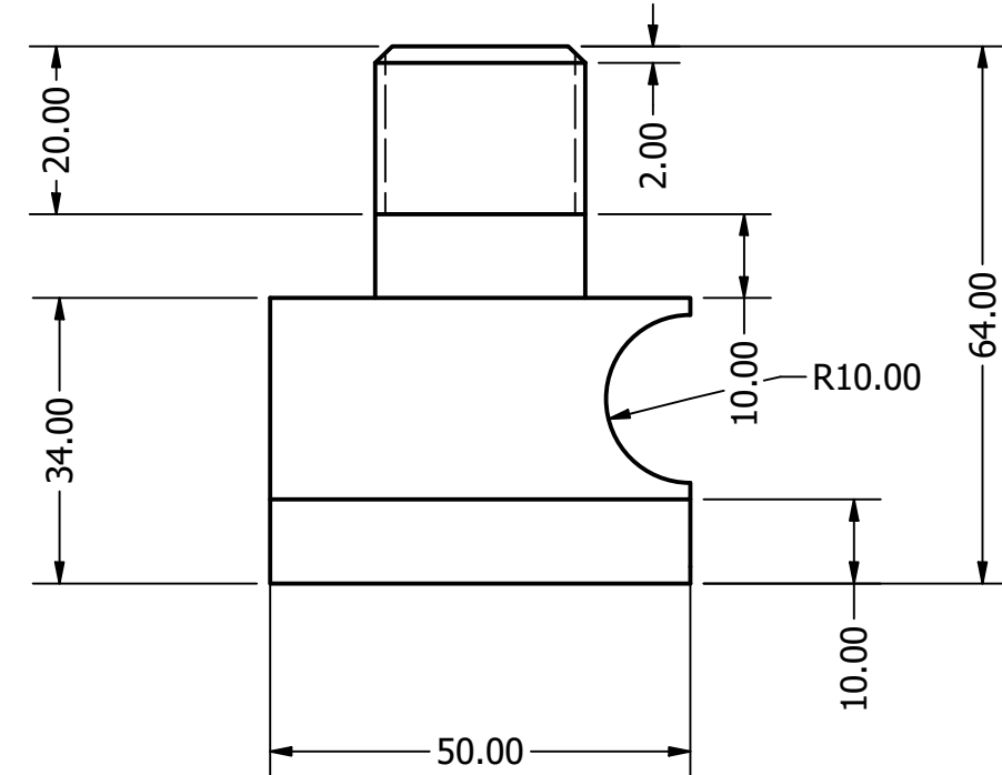
Clamp SCALE 1 : 1
