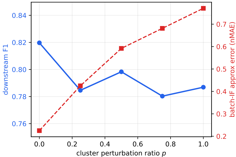
(c) Downstream F1 vs batch cohesion (ER)
