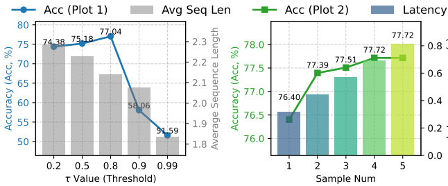
Fig. 18: Hyperparameter analysis for SPARQ 4B .
