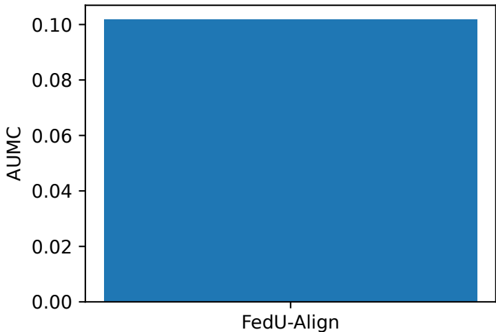
Robustness AUMC
