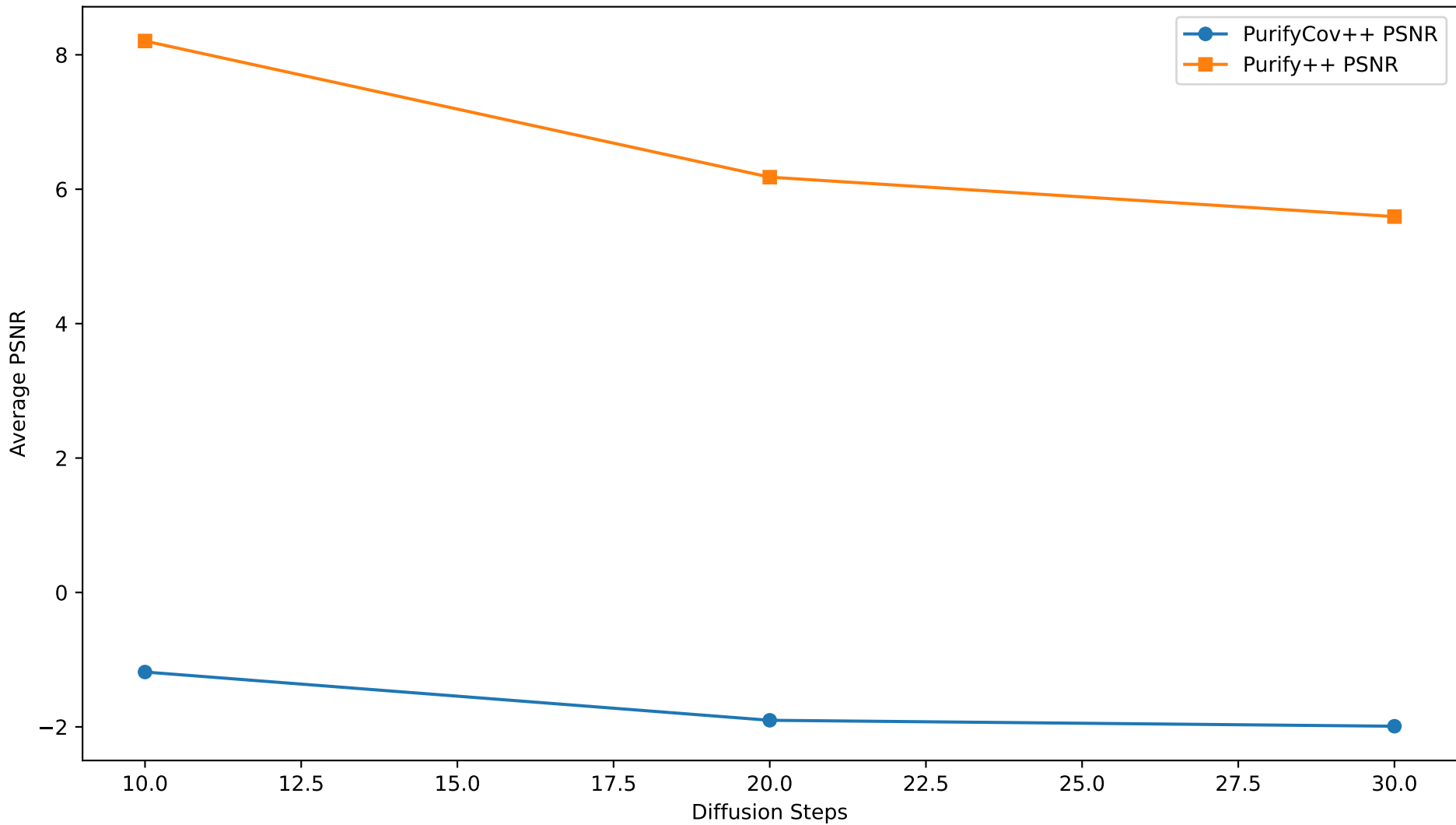
PSNR vs. Diffusion Steps
