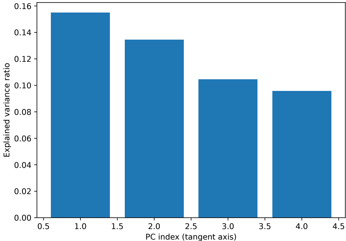
Tangent axes via PCA
