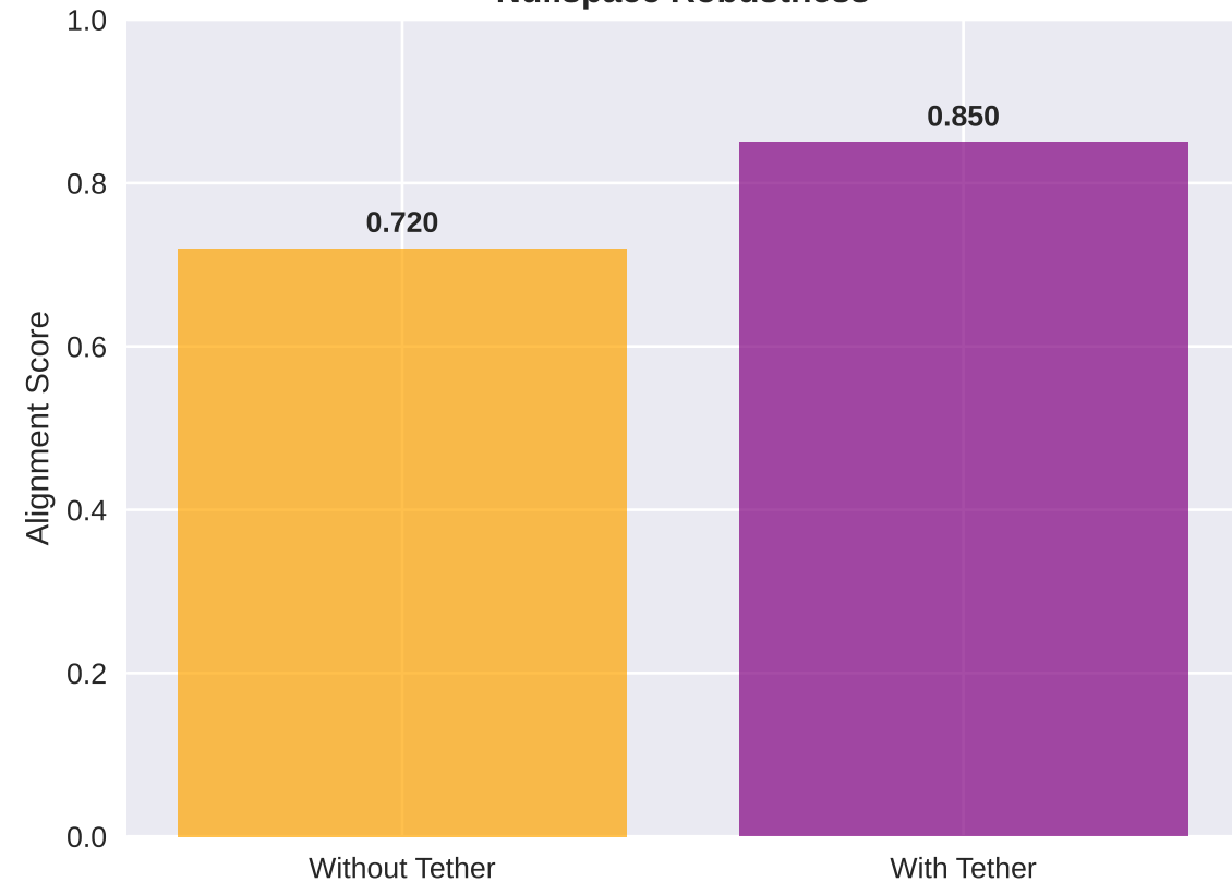
Nullspace Robustness
