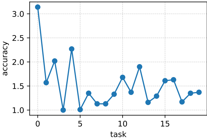
AA_lora_diffmem
