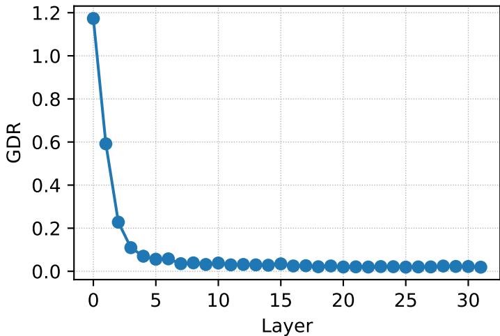
GDR - gcn
