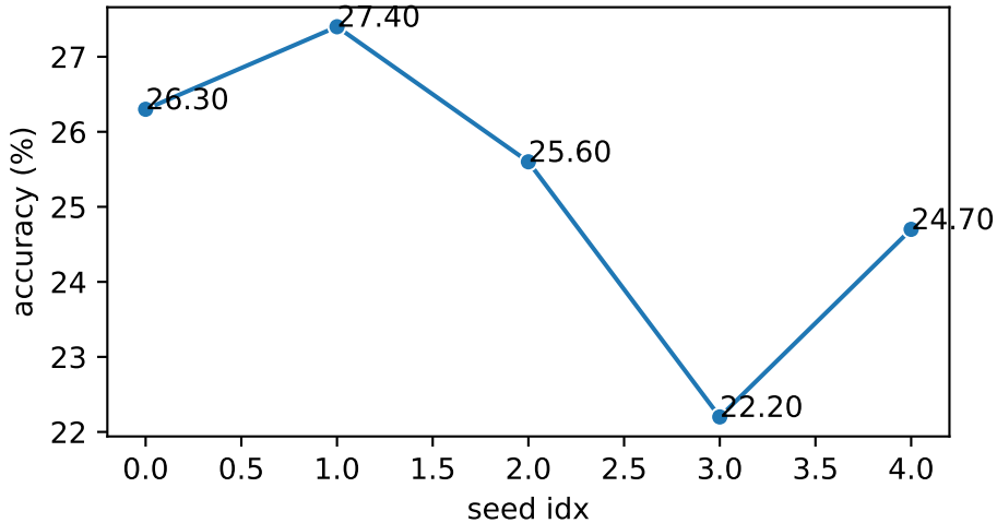
cora-gcn16
