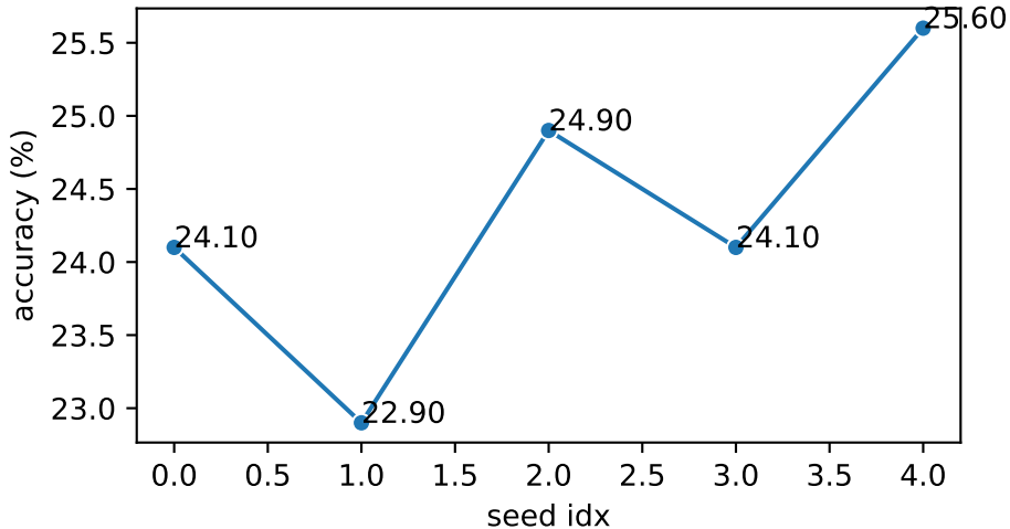
cora-gcn64
