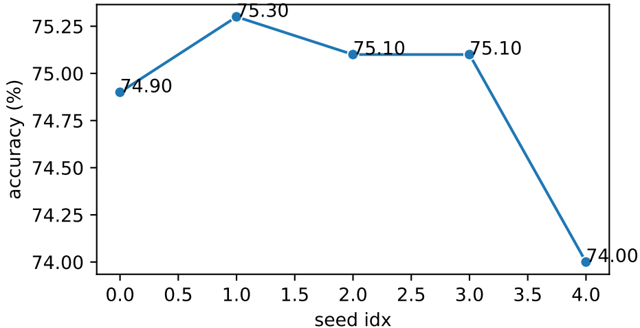
cora-gcnii64
