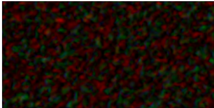
FaFT 128x256
