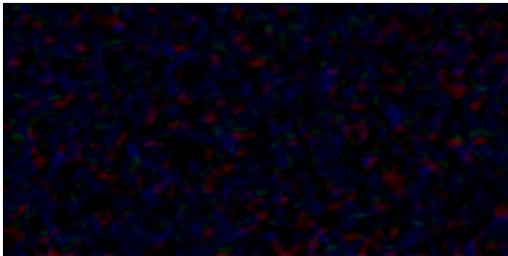
FiT 128x256
