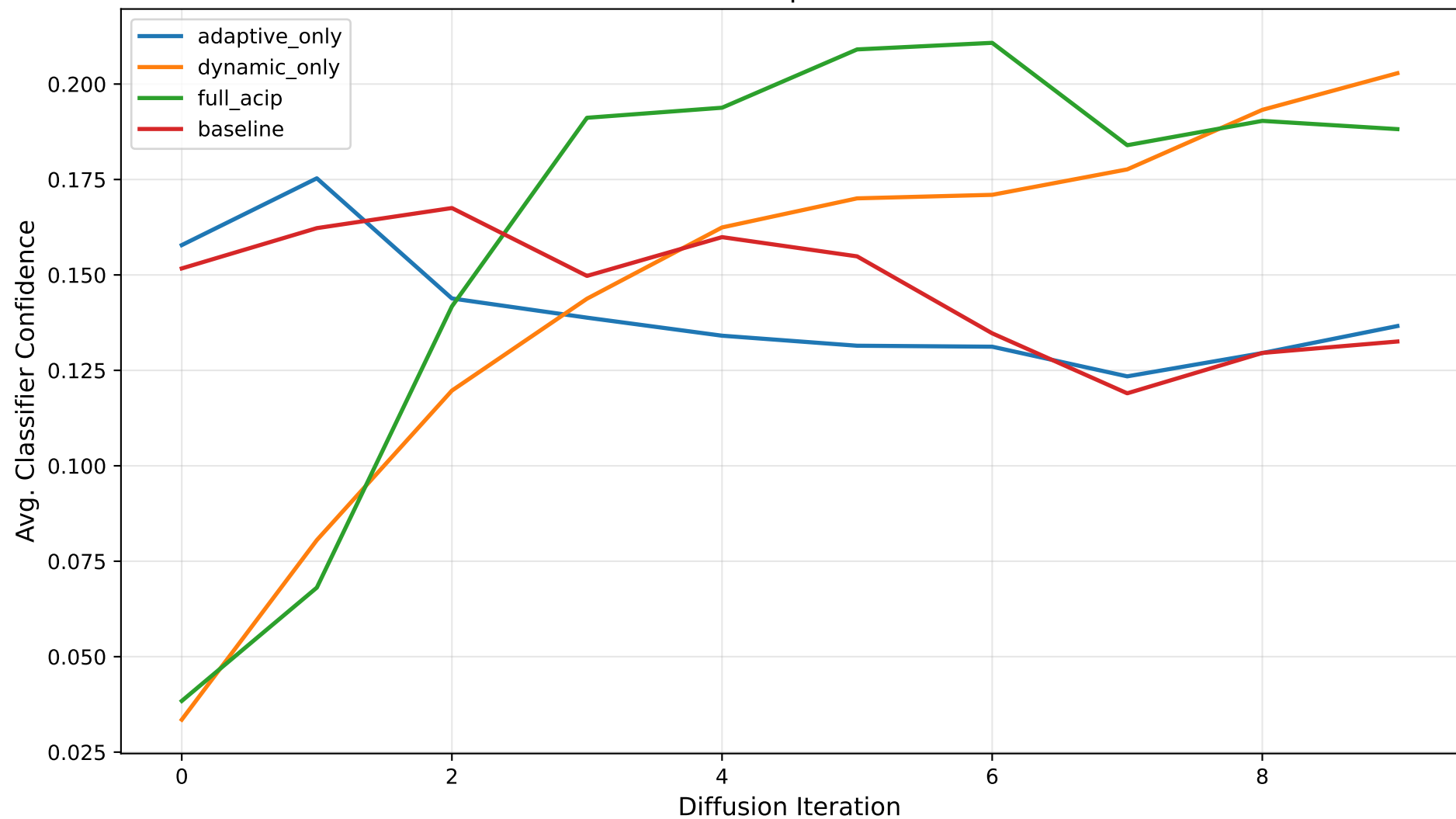
Confidence Evolution per Diffusion Iteration
