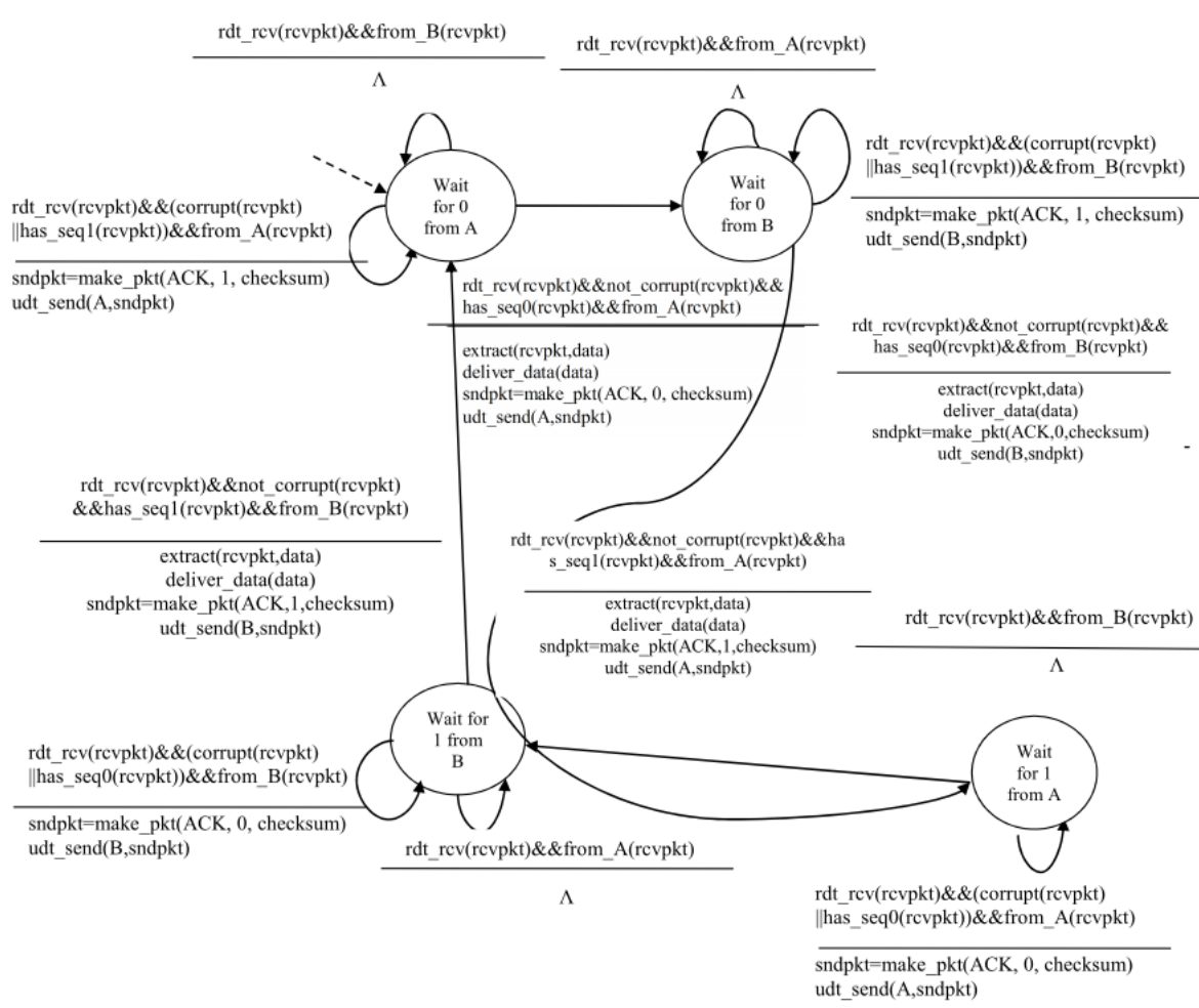
图4：3.18的接收端FSM
