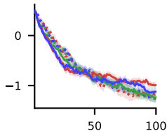
Hartmann (4D)
