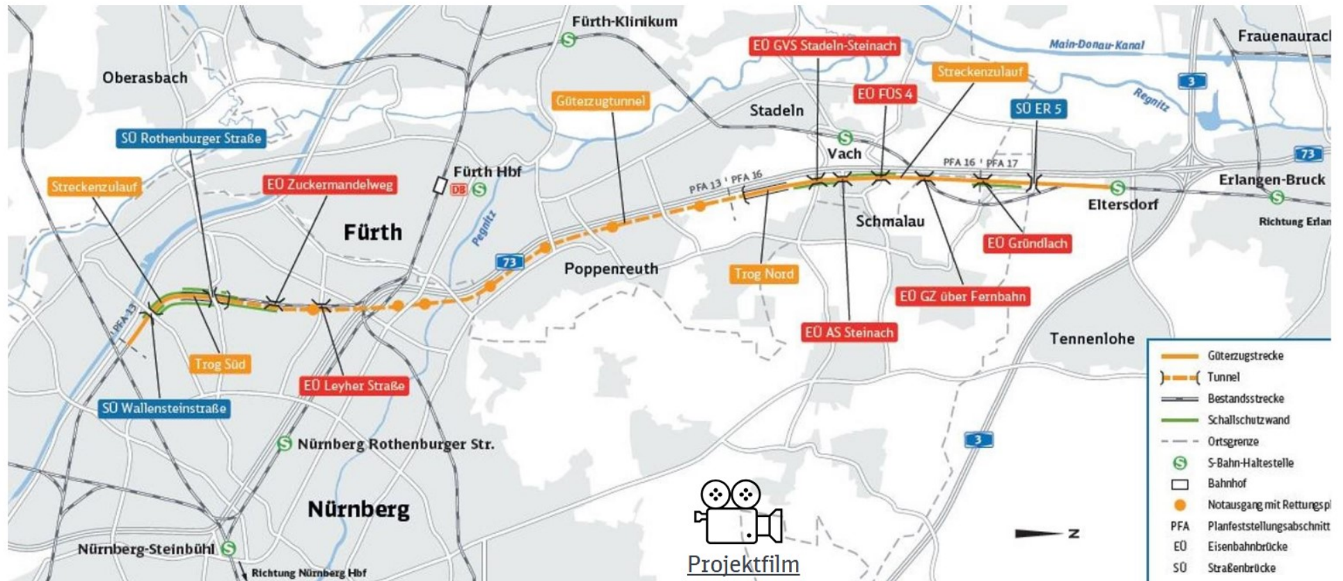
Abbildung: Lageplan – Verlauf der Güterzugstrecke Nürnberg-Eltersdorf -Teil der VDE 8.1 (Quelle: DB InfraGO AG, 2025)
