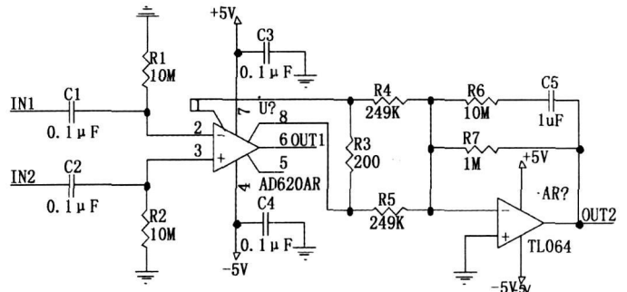
图3 隔直和初级放大电路
