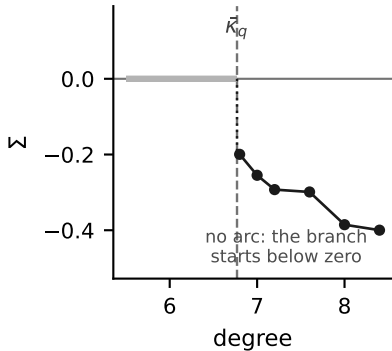
Poisson _{\Delta}
