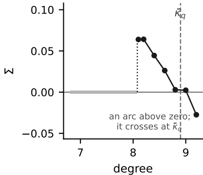
Poisson
