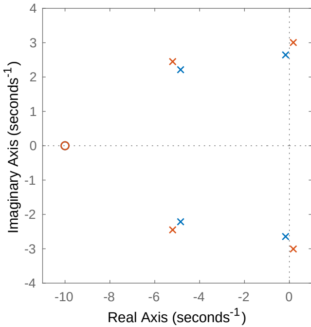
Pole-Zero Map
