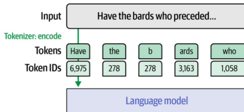
Figura 2.3: Tokenización: codificación
