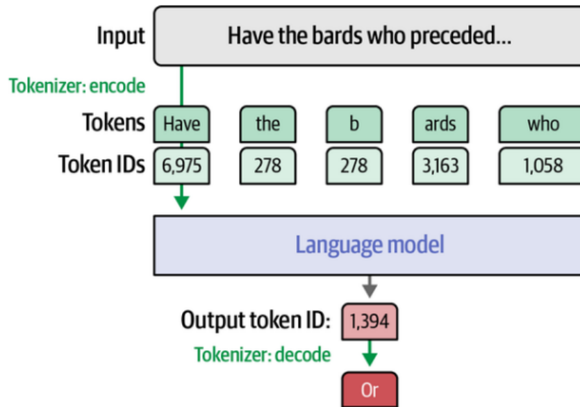
Figura 2.4: Tokenizador: decodificación
