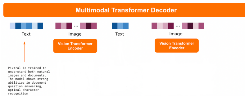
Figura 4.6: Arquitectura de Pixtral-12b
