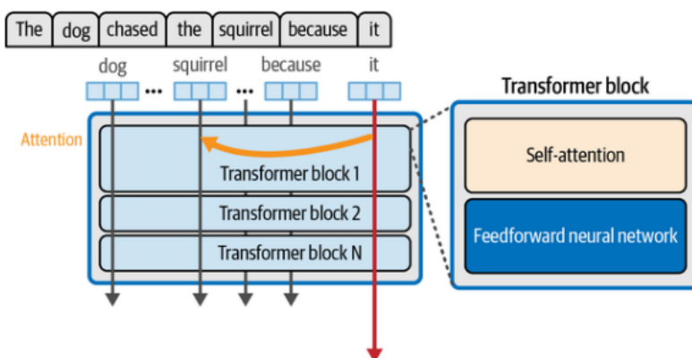
Figura 2.17: Self-attention incorpora información relevante de tokens anteriores
