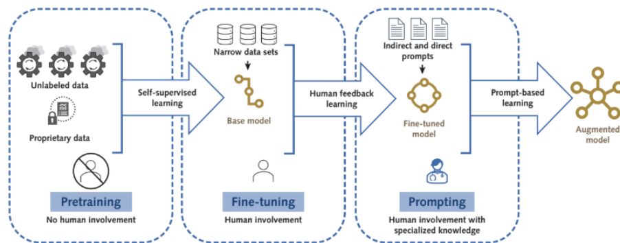
Figura 2.21: Proceso de entrenamiento para un LLM
