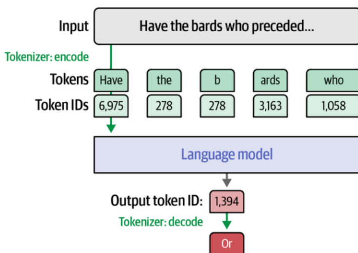
Figura 2.14: Tokenizador: decodificación
