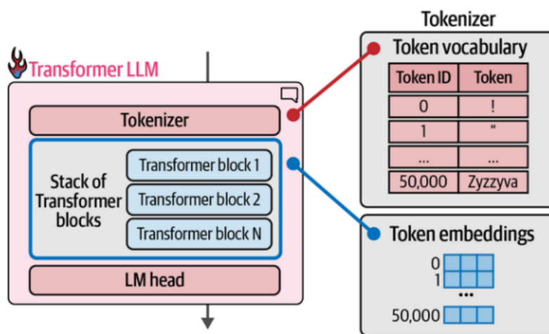
Figura 2.16: Arquitectura de un LLM basado en Transformer
