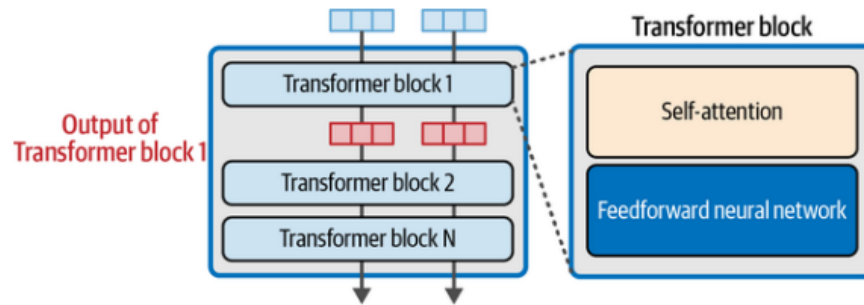
Figura 2.19: Elementos de cada bloque: self-attention y feedforward
