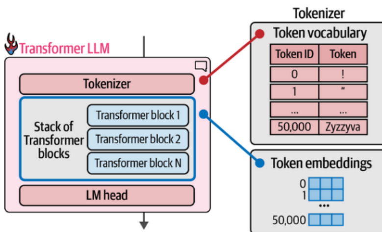
Figura 2.8: Arquitectura de un LLM basado en Transformer
