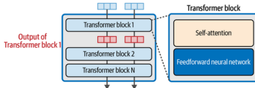
Figura 2.10: Elementos de cada bloque: self-attention y feedforward
