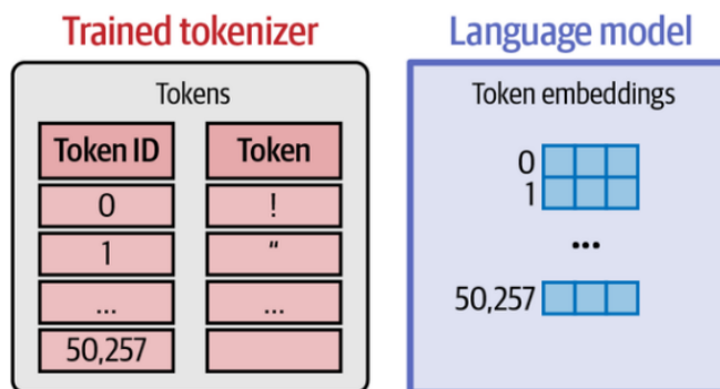
Figura 2.7: Relación entre el tokenizador y la matriz de embeddings del modelo
