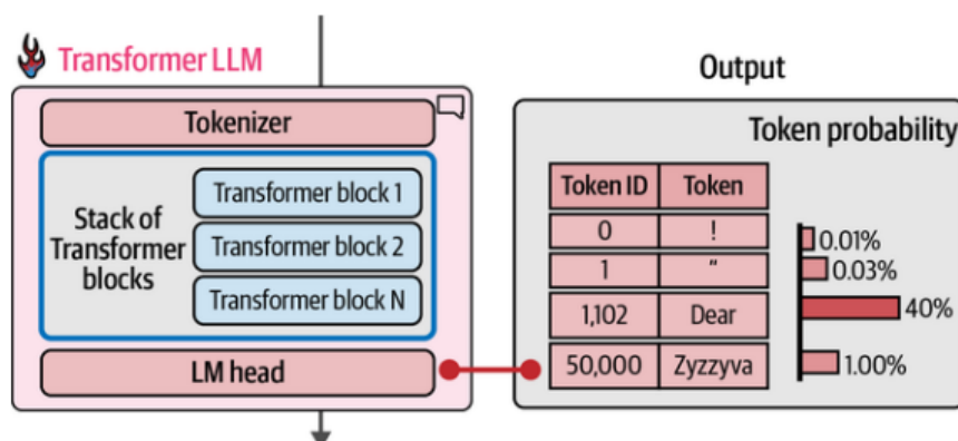
Figura 2.11: Representación del cálculo de probabilidades para cada token del vocabulario
