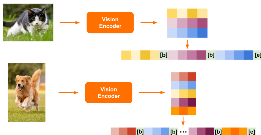
Figura 4.5: Funcionamiento del codificador de visión
