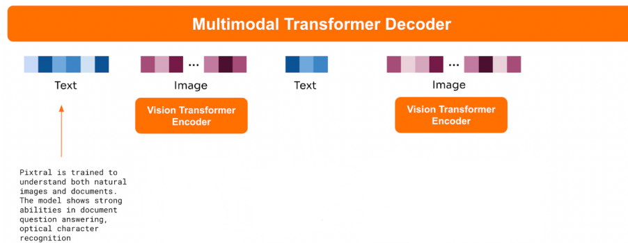
Figura 4.6: Arquitectura de Pixtral-12b
