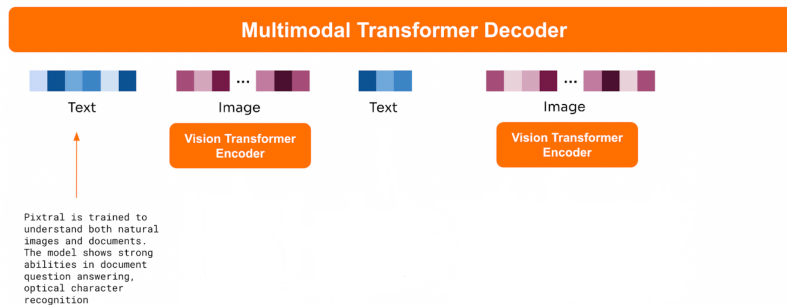
Figura 2.29: Arquitectura de Pixtral-12b
